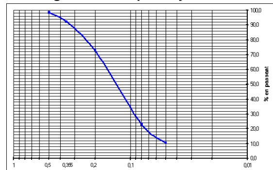
Courbe granulométrique moyenne :
